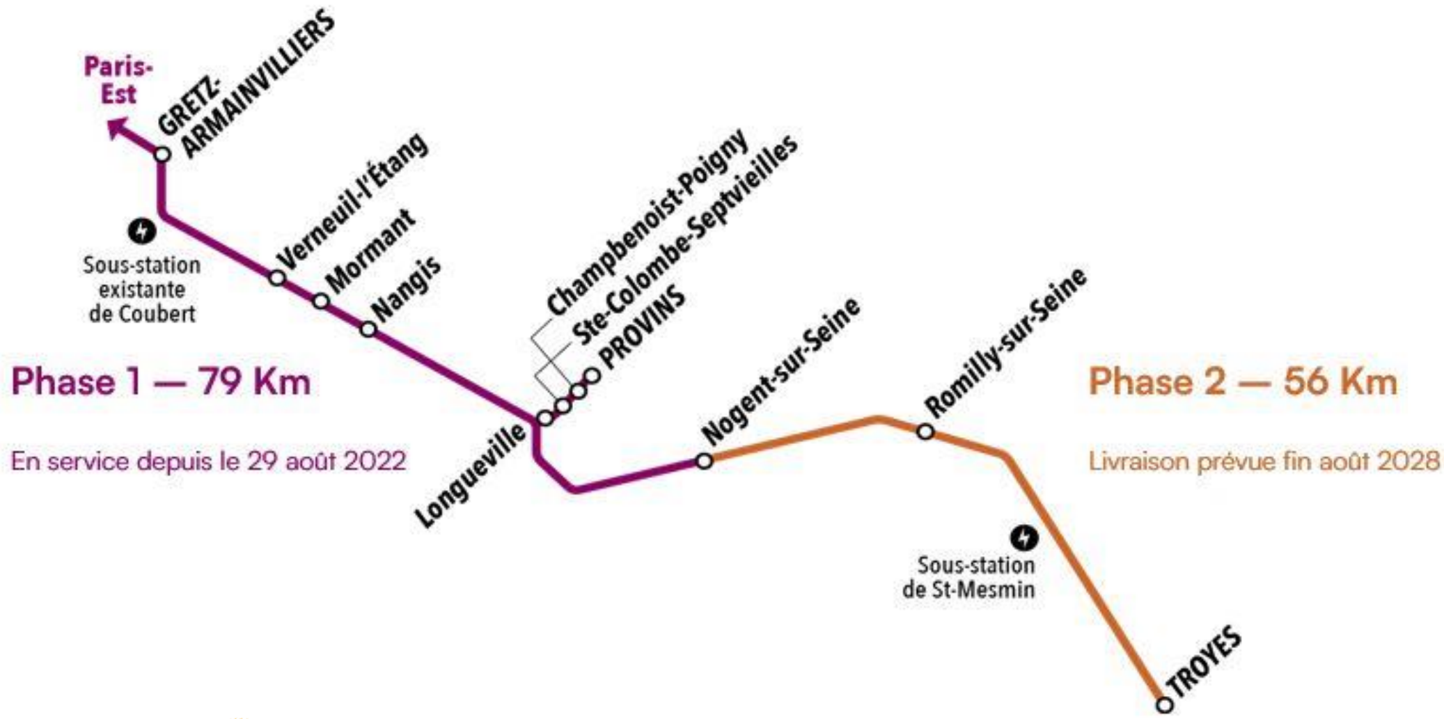
Le projet d'électrification de la ligne Paris/Troyes
