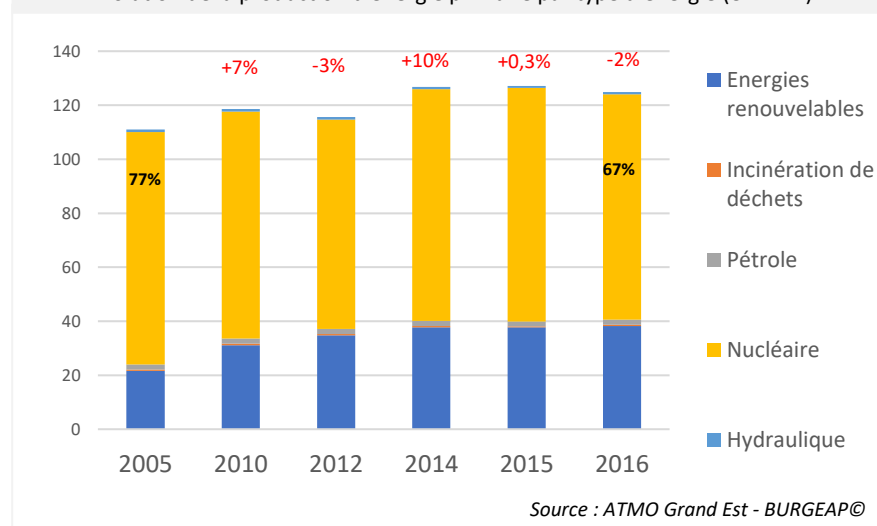
Evolution de la production d'énergie primaire par type d'énergie (en TWh)
